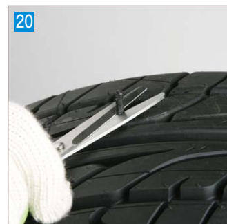
20 タイヤの外側に出たゴムを、1ミリから1.5ミリ残して切り取る
