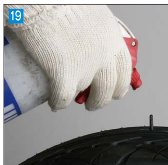
19 エアーを入れ、霧吹きスプレーでエアームれをチェックする
