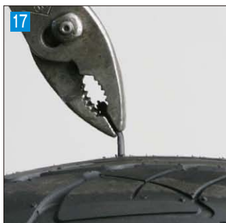
17 タイヤの内側を手で押さえ、外側に出たゴムを引っ張り、プラグパッチを密着させる
