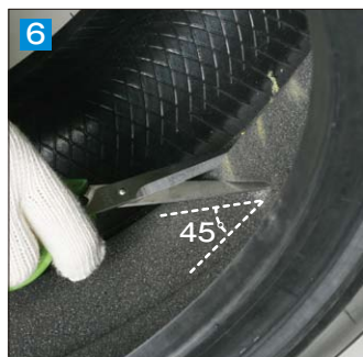
6 ハサミを使い、特殊吸音スポンジの凸部に斜め(45度位)に2ヶ所切れ込みを入れる ※作業にカッターは絶対に使用しないでください
