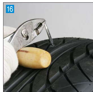
16 ドライバーの柄をテコにして、タイヤの外側に出た金属部分をプライヤーベンチで引き抜く
